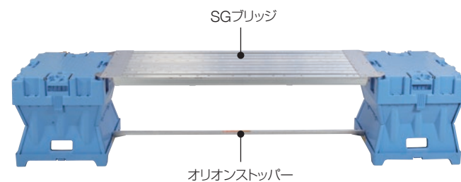
オリオンストッパー<下部連結棒> 長さ:1510mm 質量:600g
