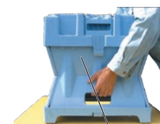
3 側板小と側板大がしっかりかみ合っていることを確認しながら側板大と底板とのロックを必ず固定します。側板大の凸部が表から見えるまで押し込んでください。
