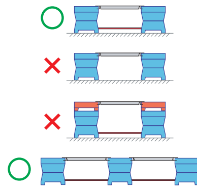
下段を組み立てた状態、上段も組み立てた状態での組み合わせ
